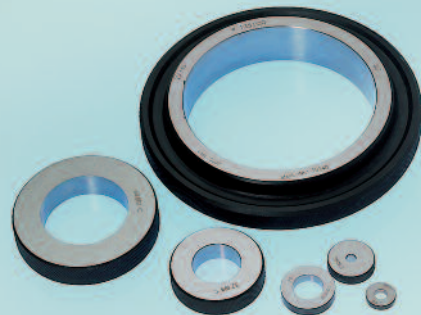
Einstellringe nach DIN 2250
